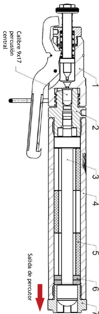
Fig. : Pistola de sacrificio de ganado Blitz Schlag (no tensada)
